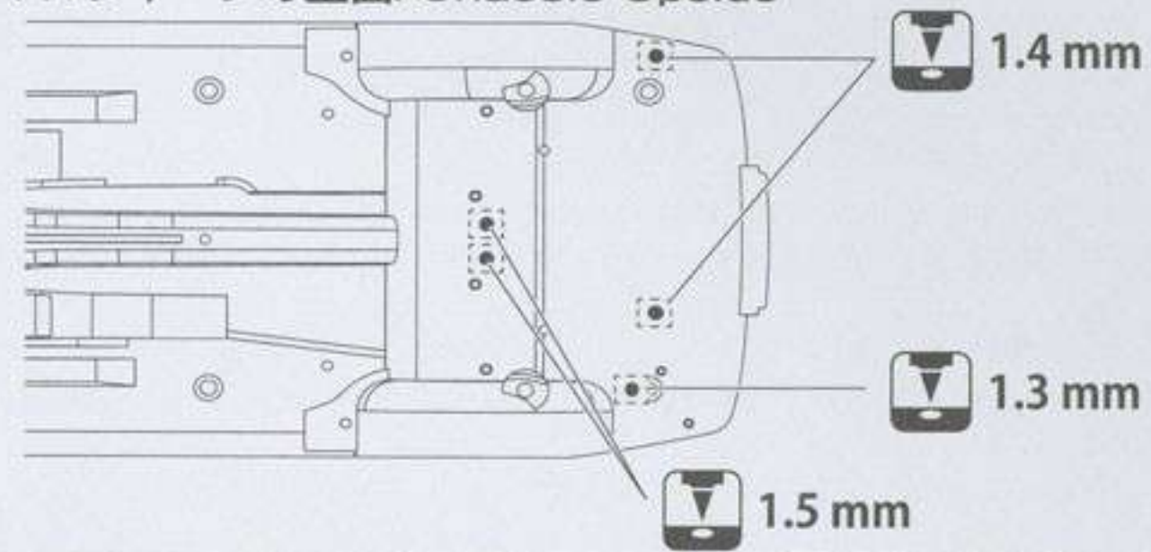
A1シャーシの上面/Chassis Upside
